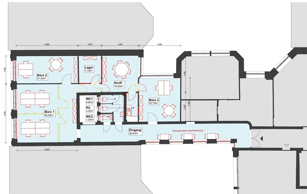
Grundriss Ballindamm 13, Variante B
