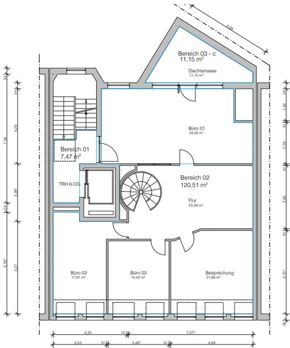
Grundriss 6. OG
