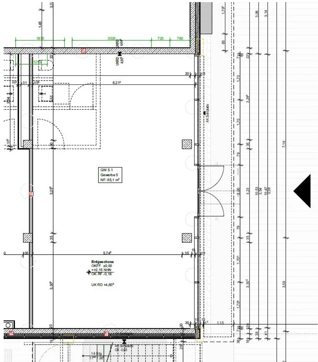
Grundriss Gewerbe5
