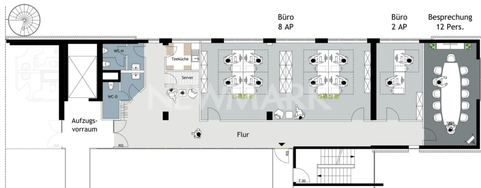
4. Obergeschoss, ca. 223 m 2
