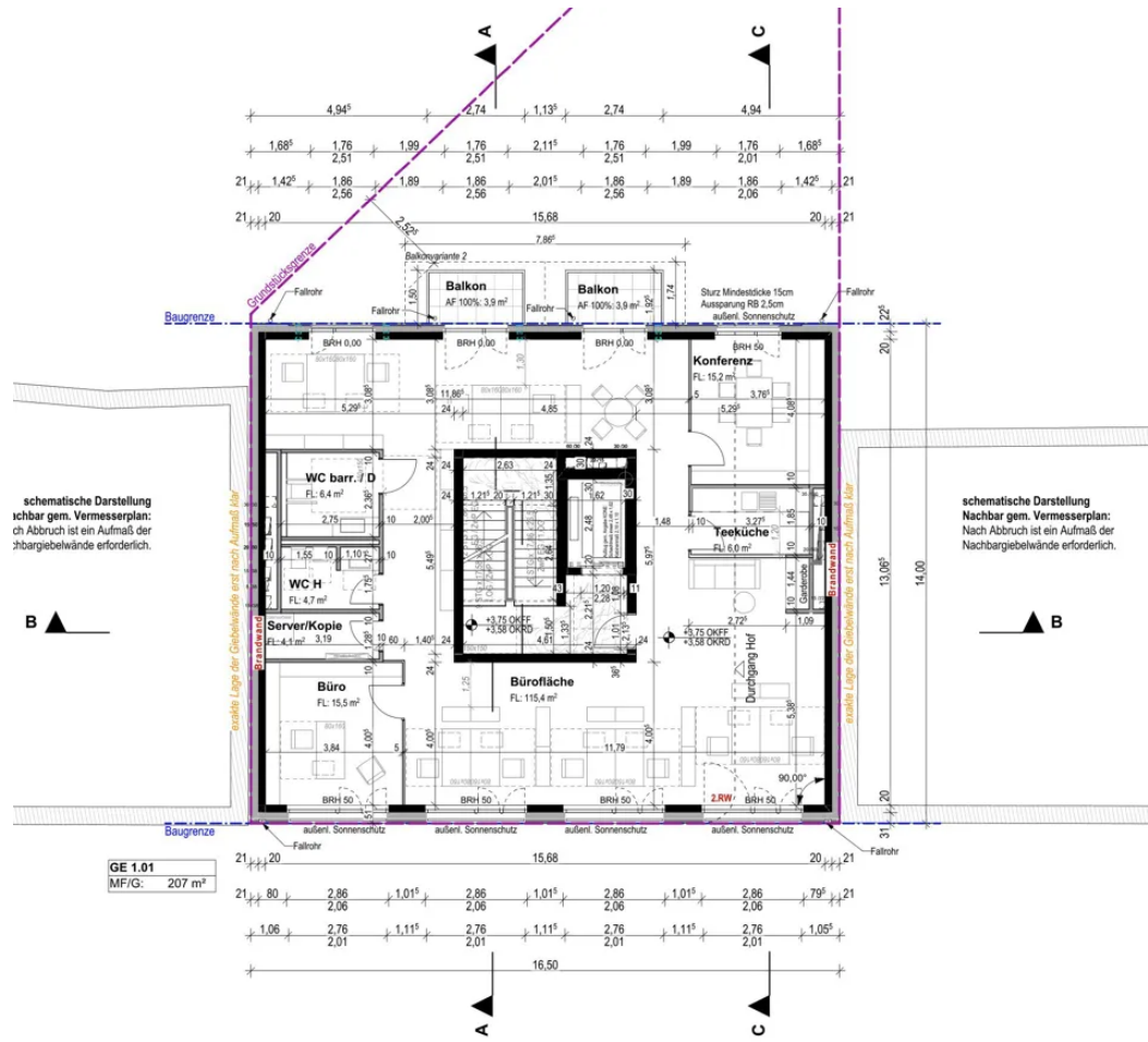
Grundriss 1. Obergeschoss
