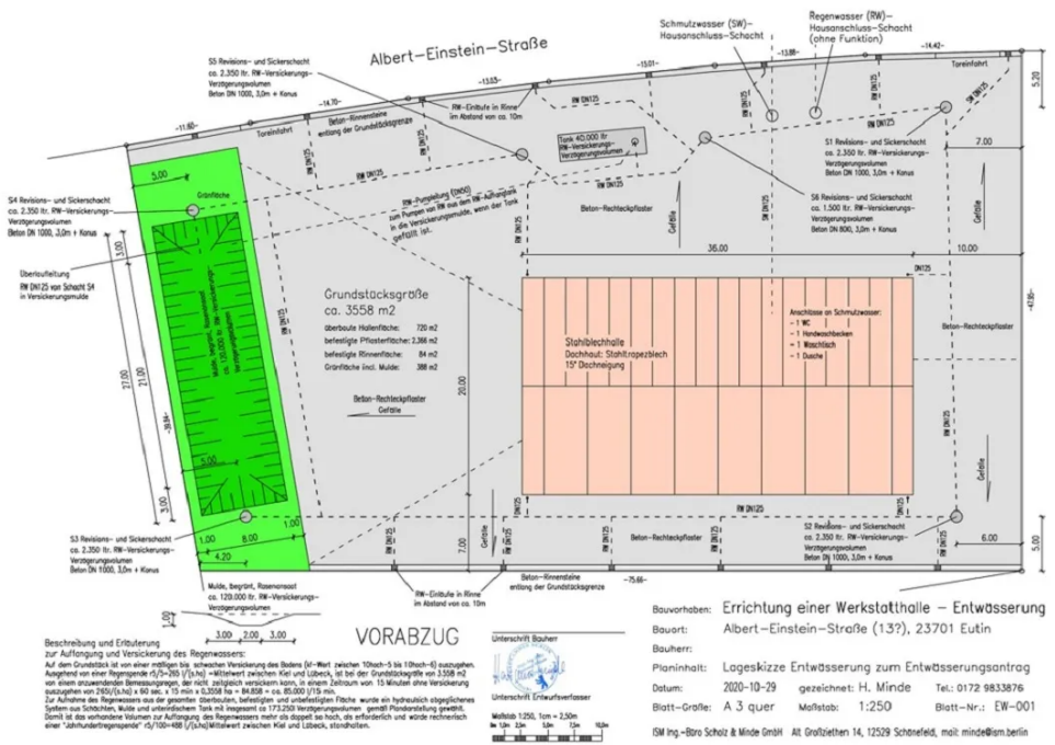
Grundriss
