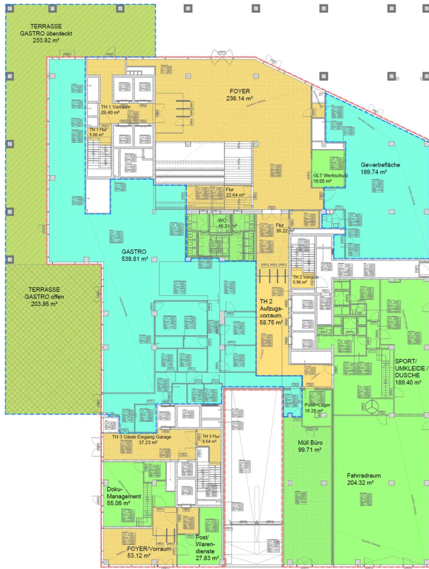
Grundriss: EG
