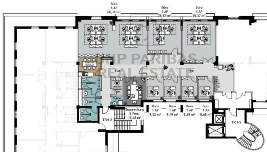
Grundriss - 6. Obergeschoss
