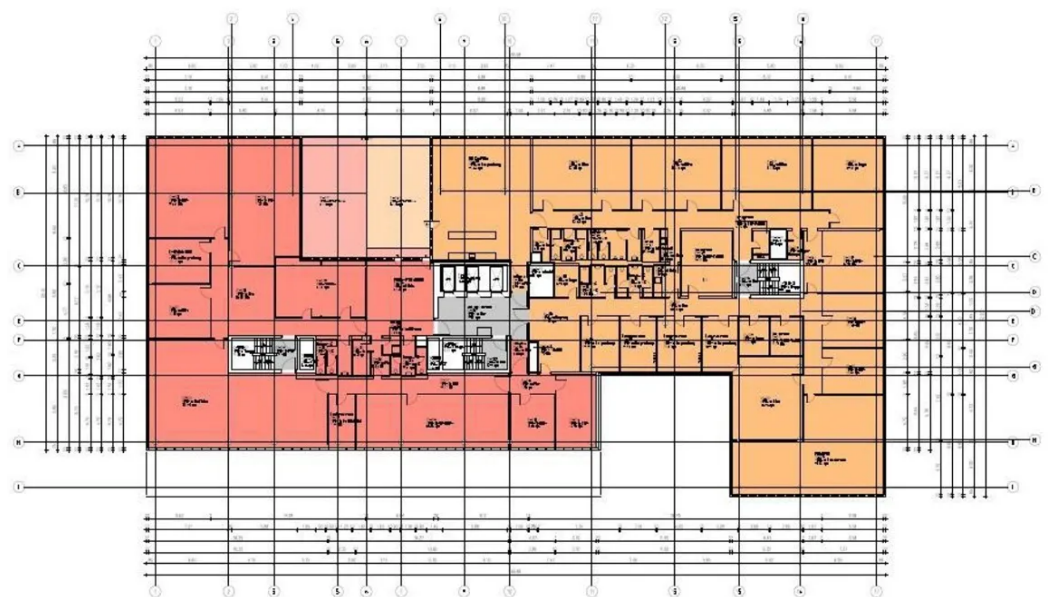
Grundriss OG 1, 1698 m 2
