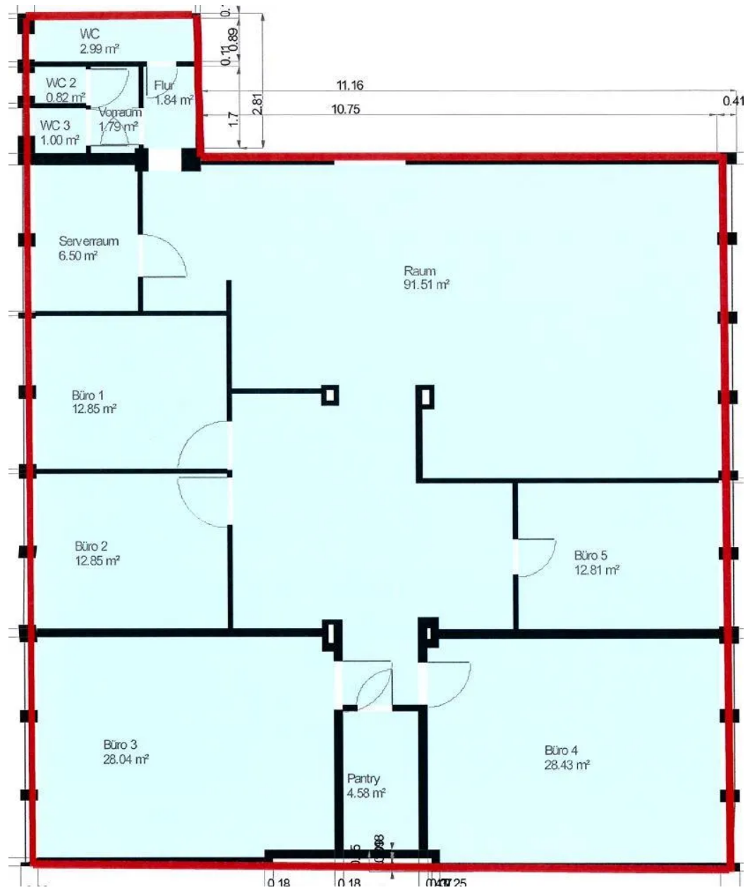
Grundriss 1. Obergeschoss
