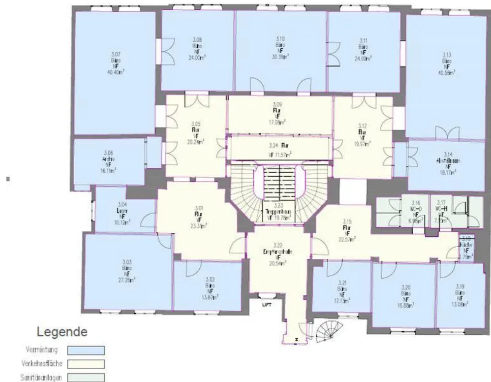
Grundriss 3. Obergeschoss
