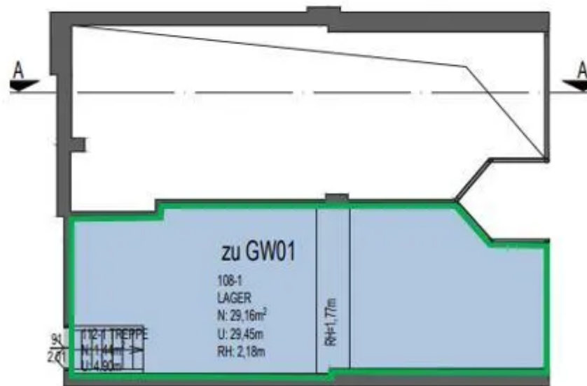
Grundrisse MZ
