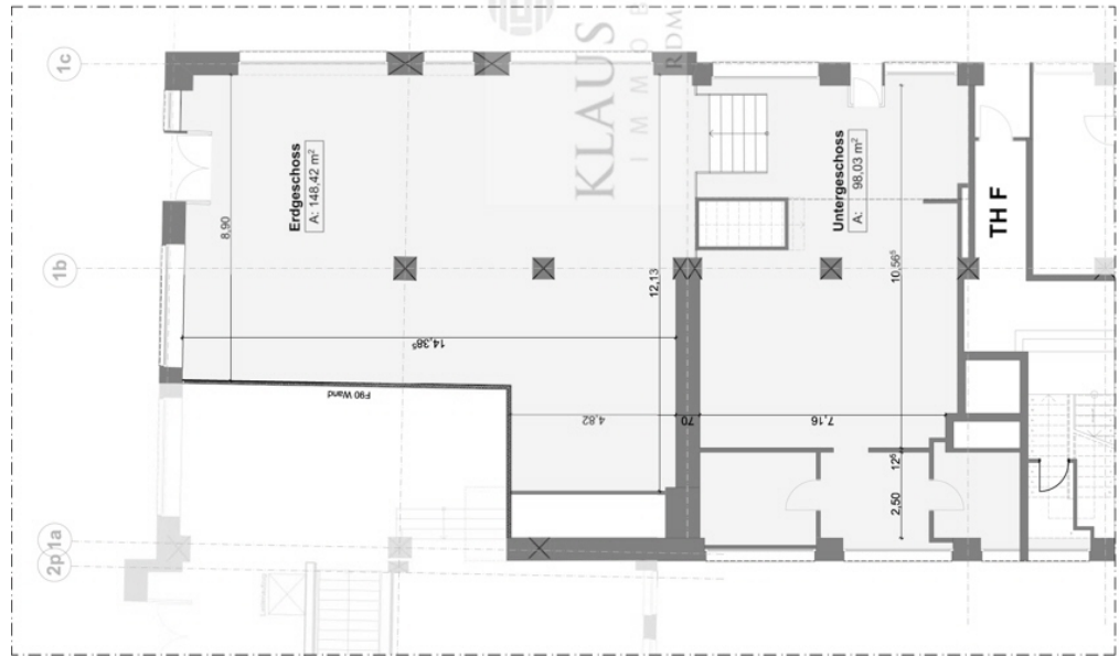
Grundrisse
