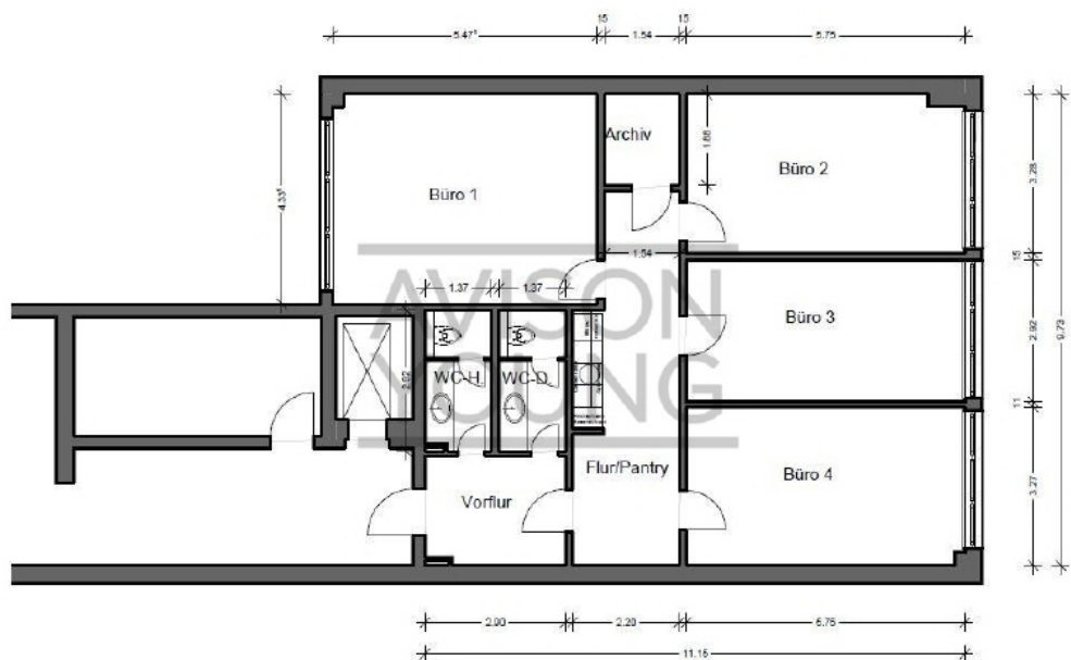
3 OG
