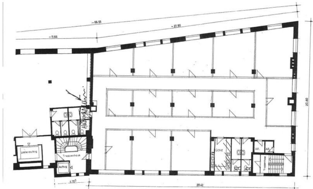
Gruendriss 4 Obergeschoss
