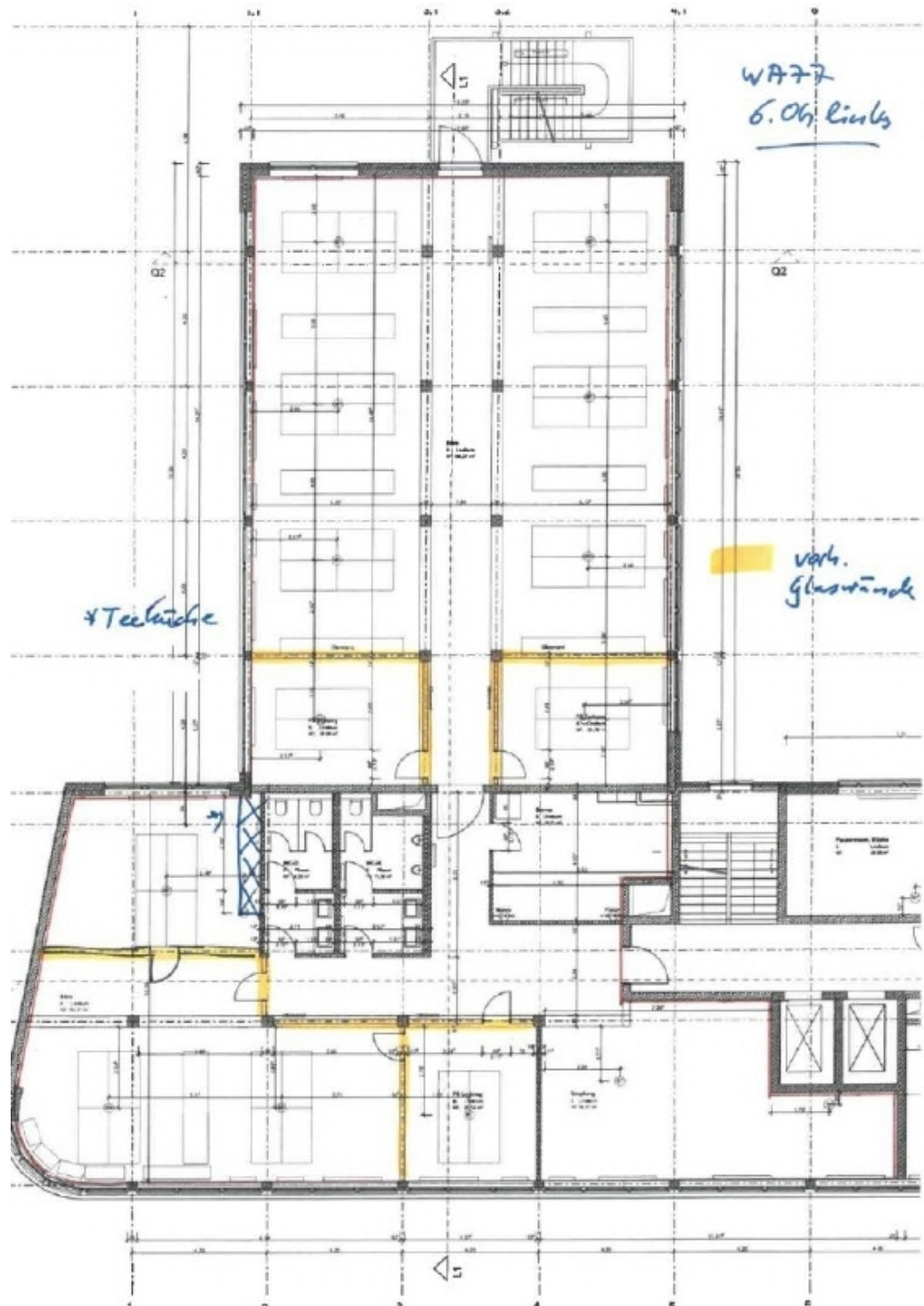
Grundriss 6 Obergeschoss
