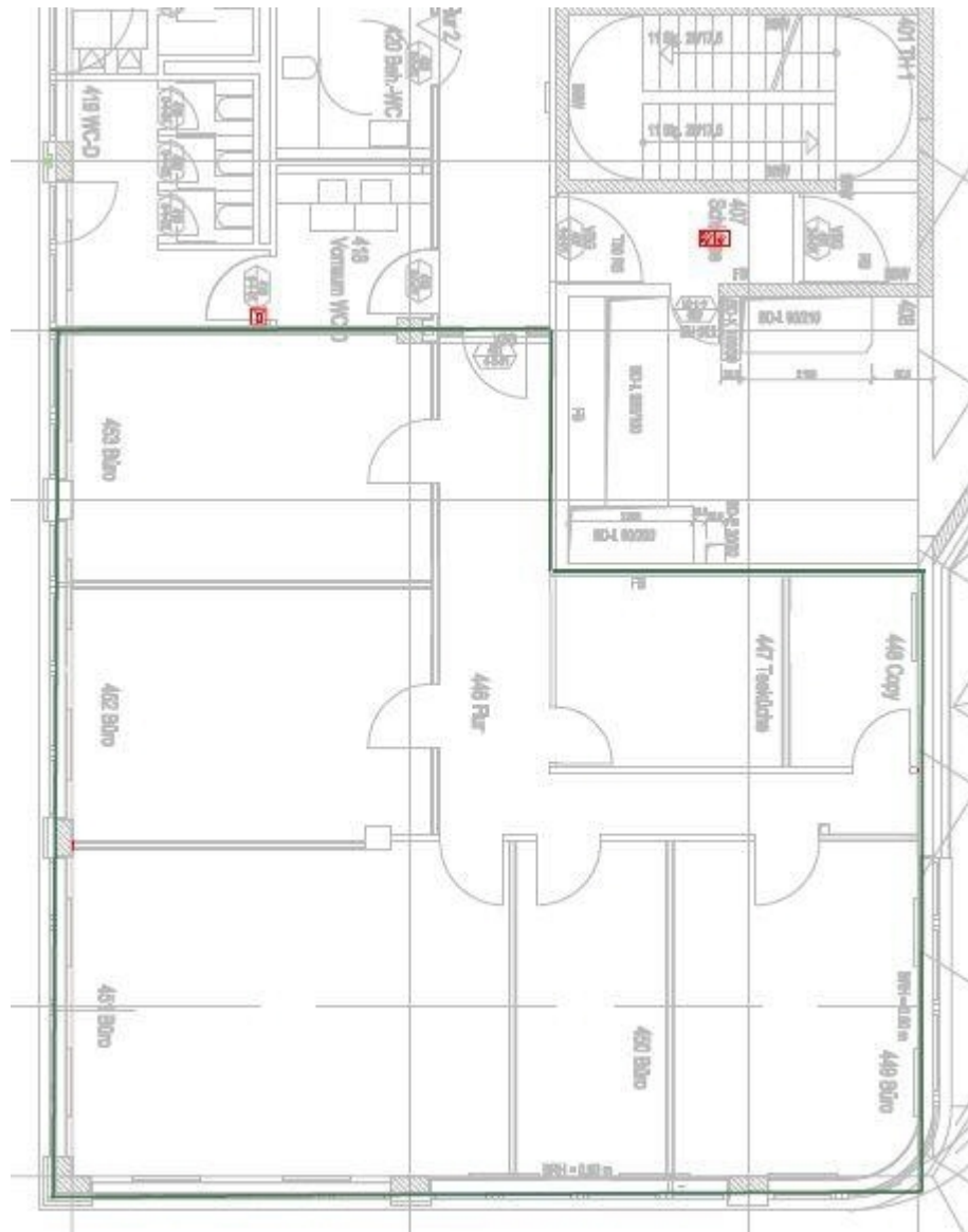
Grundriss 4Obergeschoss
