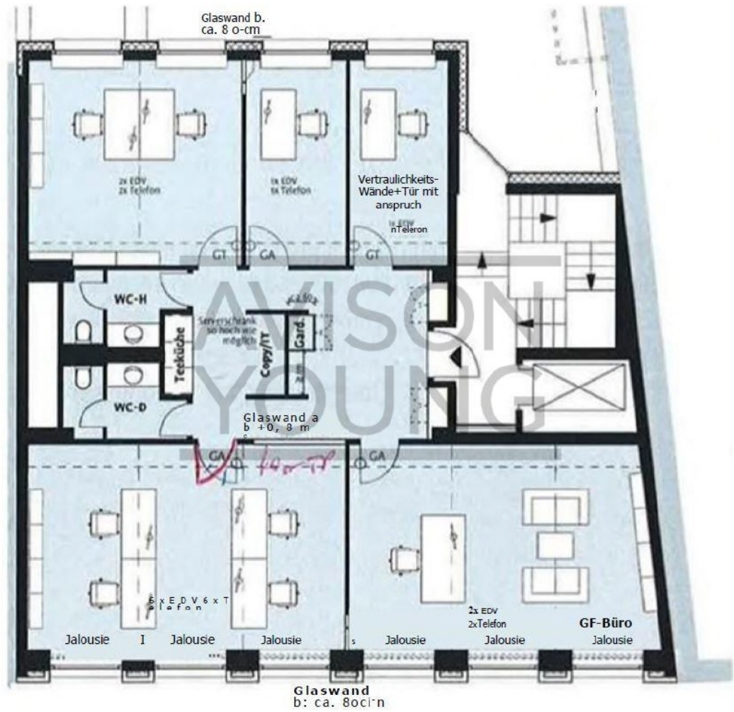
6. Obergeschoss mit ca. 156 m²
