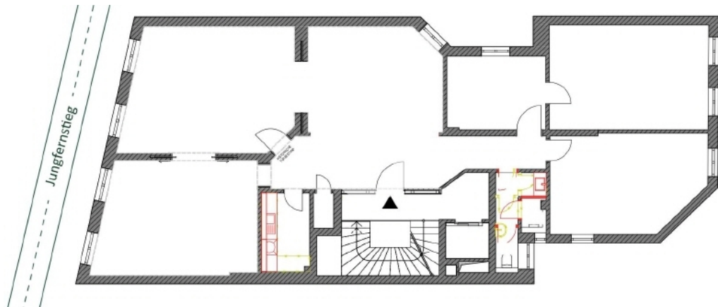
4 Obergeschoss mit ca 194 m 2 - Bestand
