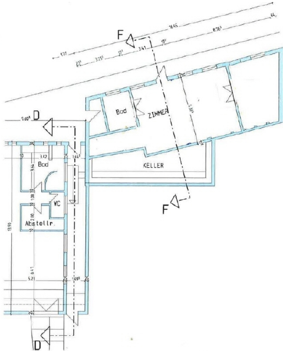
Grundriss Wohnbüro
