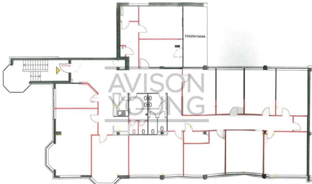
1. Obergeschoss
