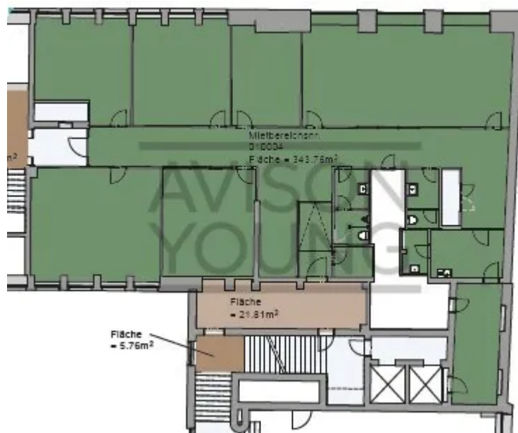
Hochparterre mit ca. 392 m²
