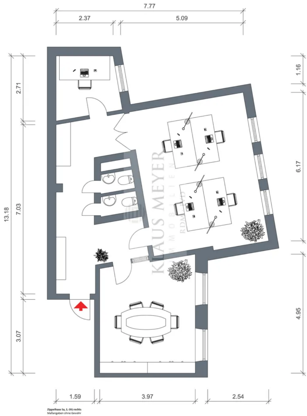
Z5a 5a, 145m² Basisebene
