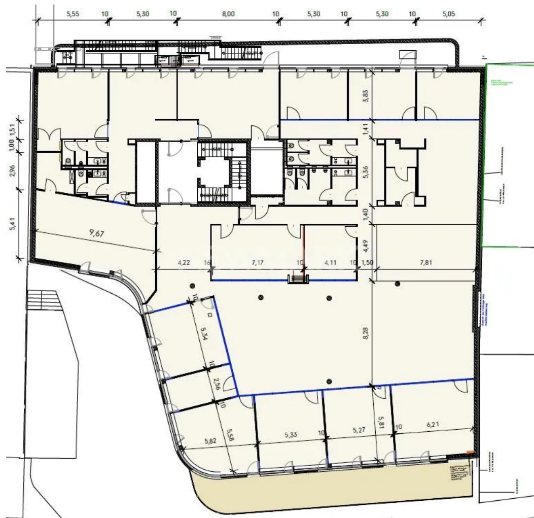
1. Obergeschoss, ca. 931 m 2
