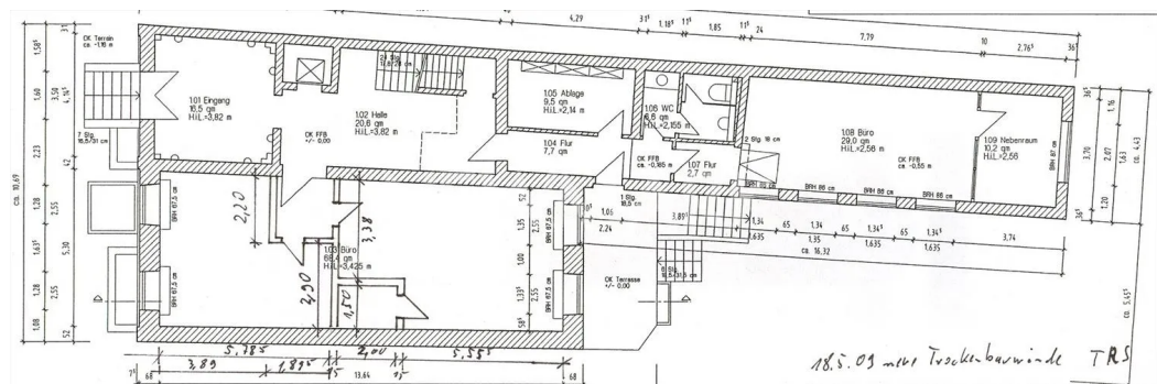
Grundriss Erdgeschoss
