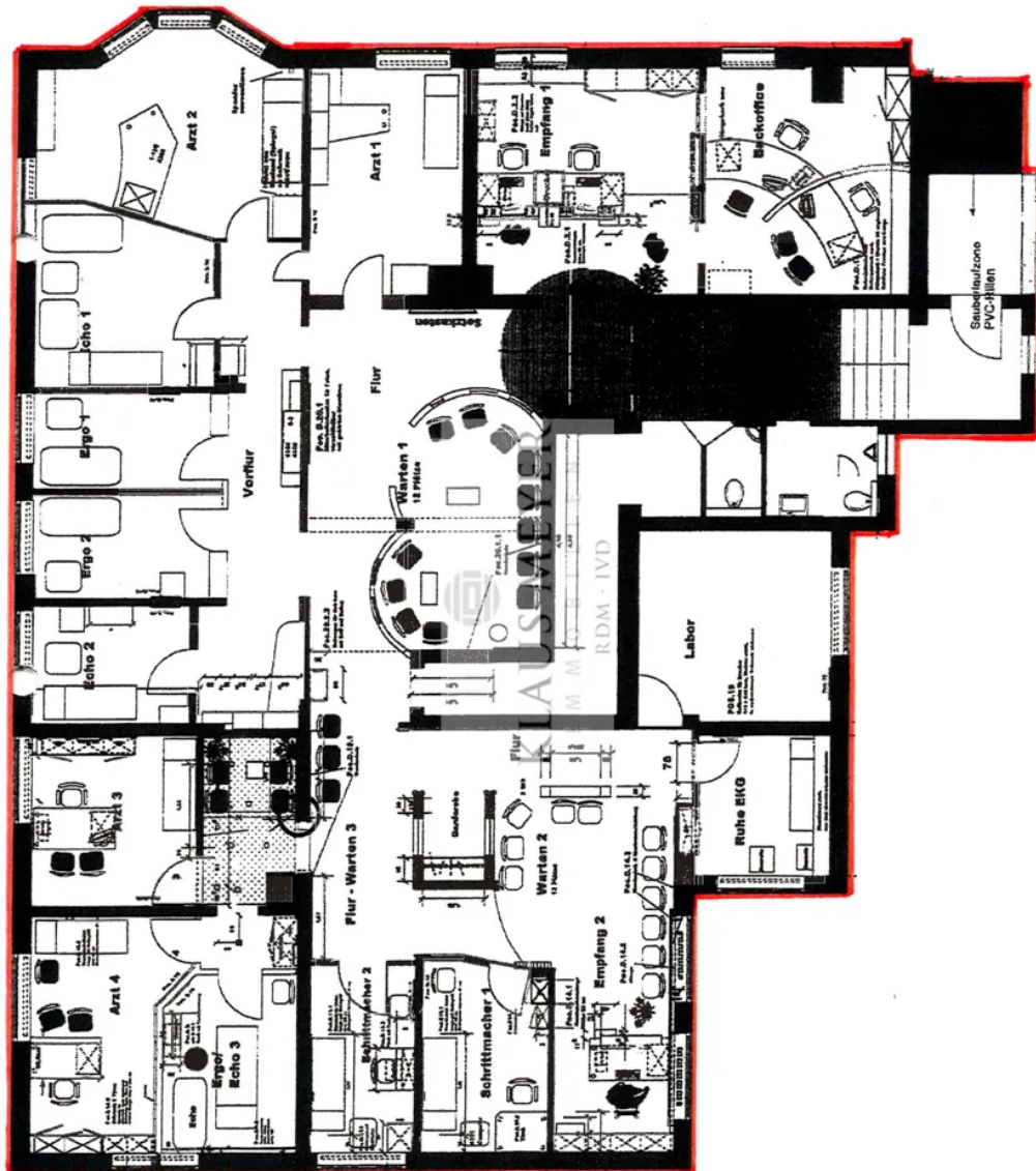
Hochparterre
