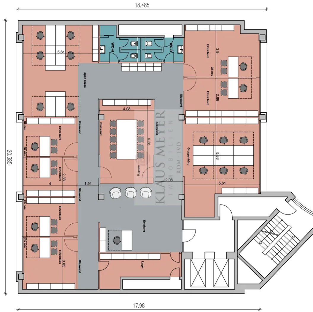
6.OG, Planungsidee
