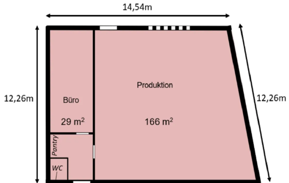
Grundriss
