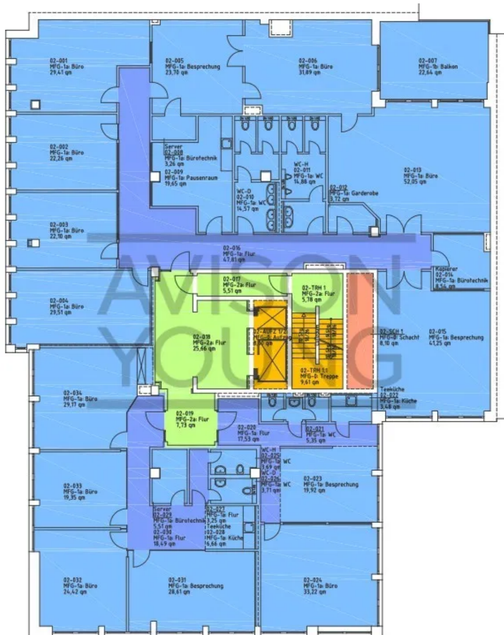
2. OG | 559 m 2
