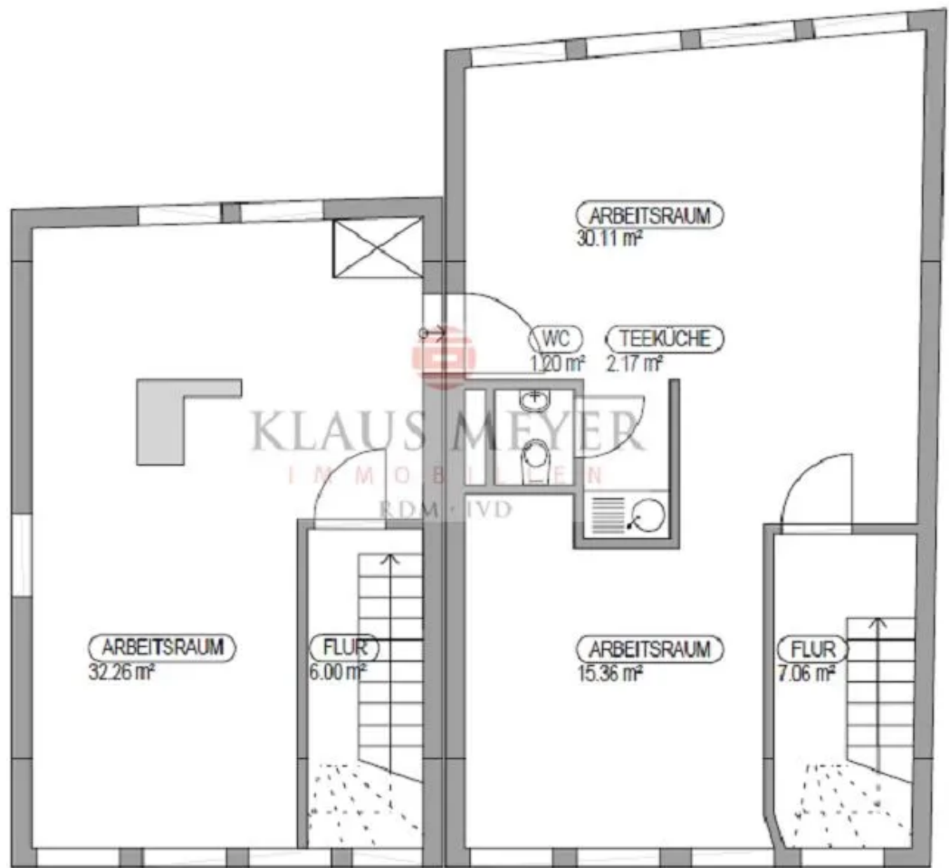
Grundriß 2. OG
