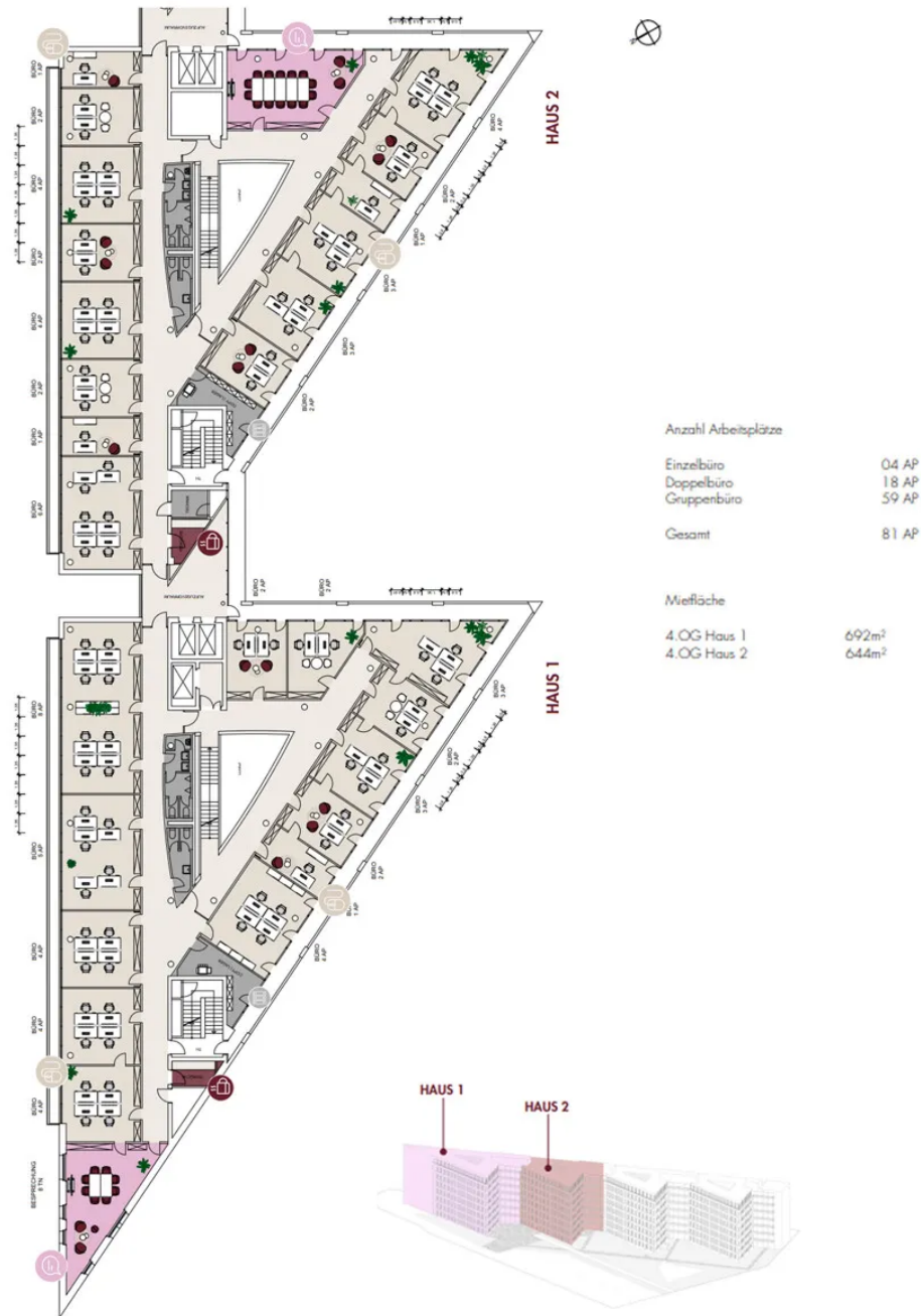
Grundriss 4. OG
