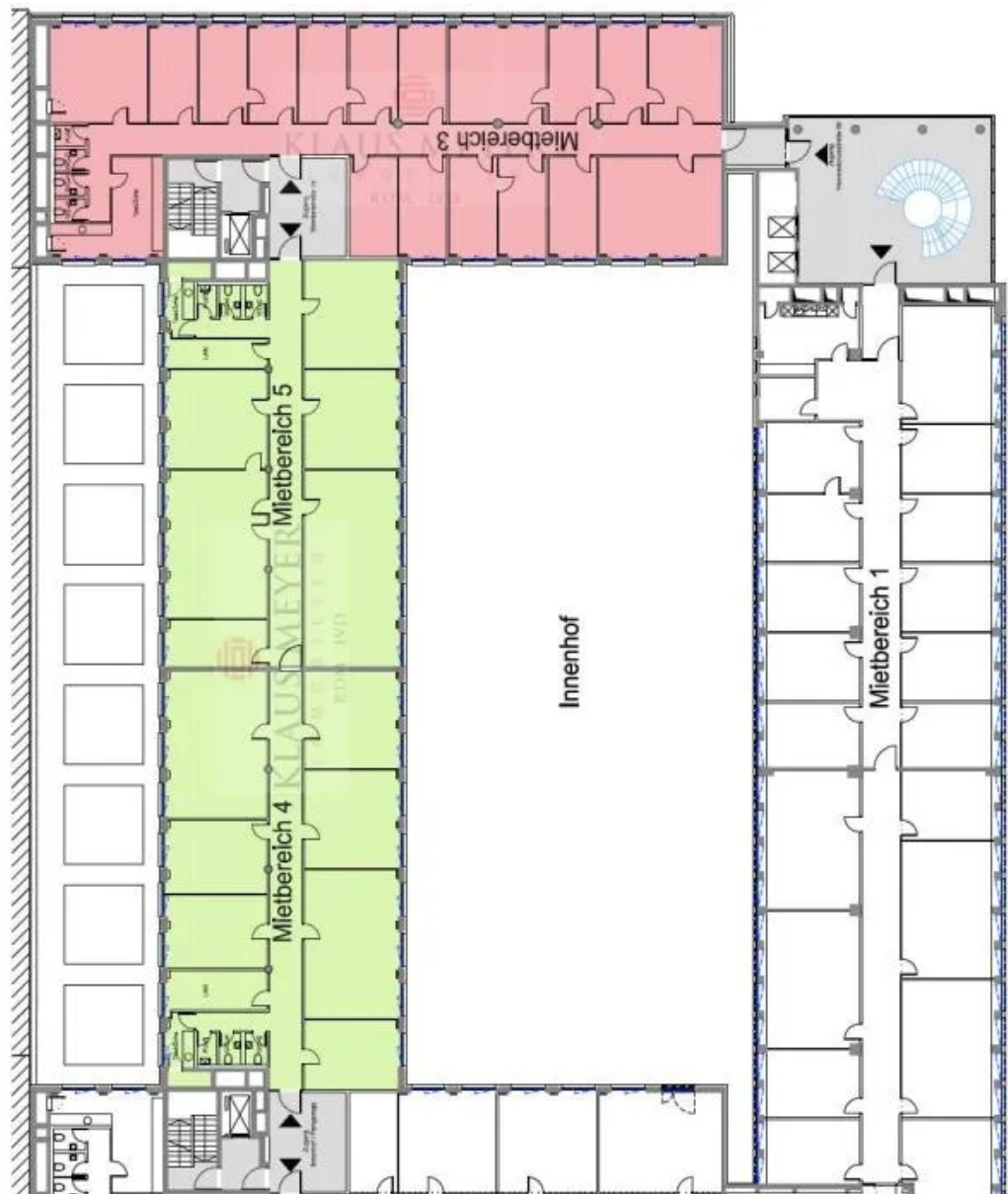
Grundriss
