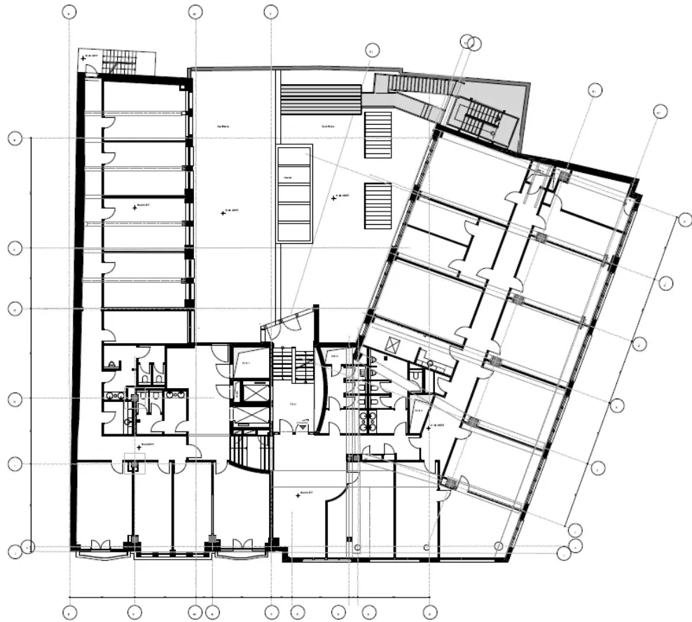
3. Obergeschoss, ca. 843 m 2
