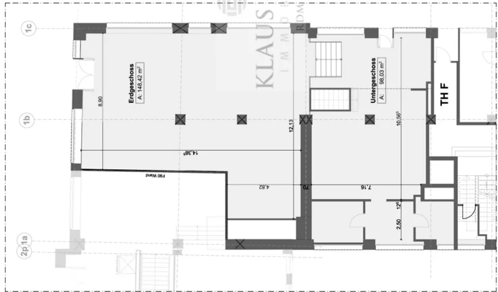
Laden Grundriss
