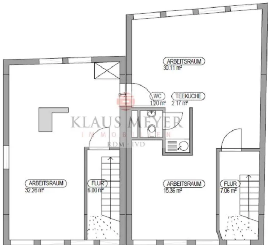
Grundriß 2. OG
