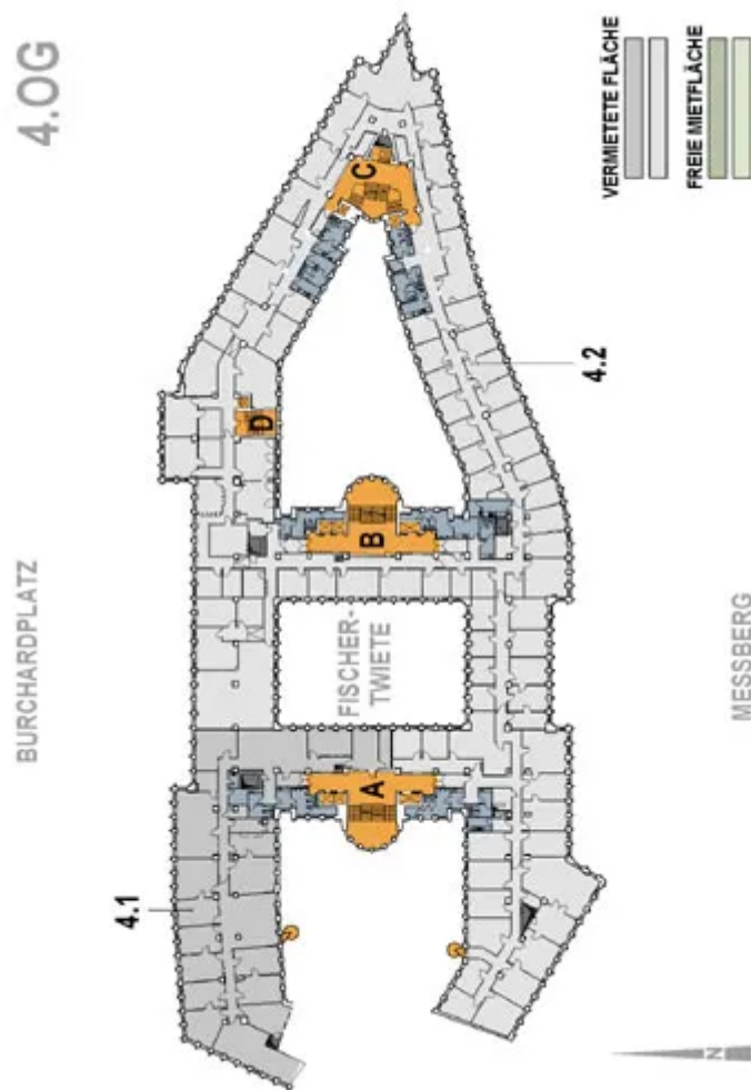
Chilehaus Etagengrundriss
