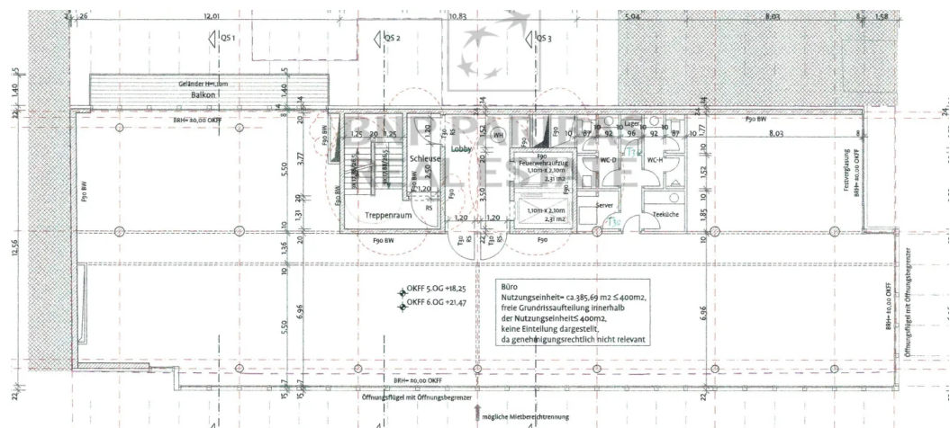
Grundriss - 6. Obergeschoss
