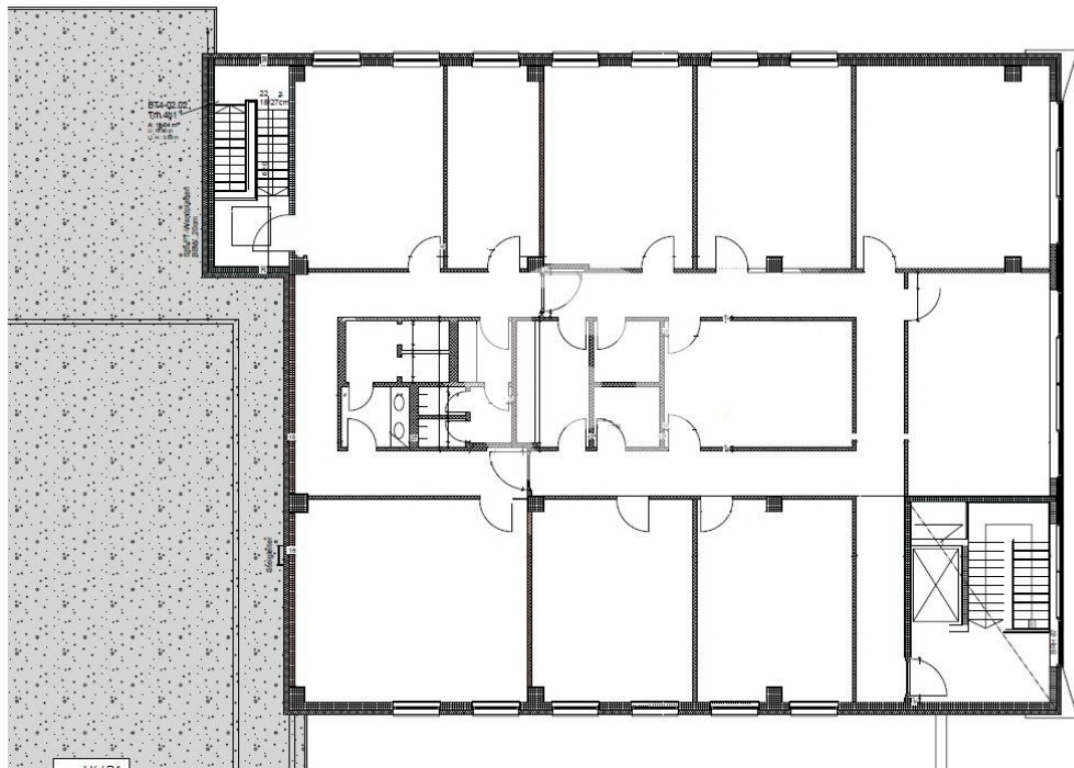
Haus B - 1. Obergeschoss mit ca. 484 m 2
