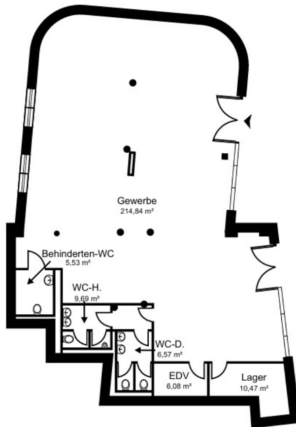
Grundriss EG, ca 253 qm
