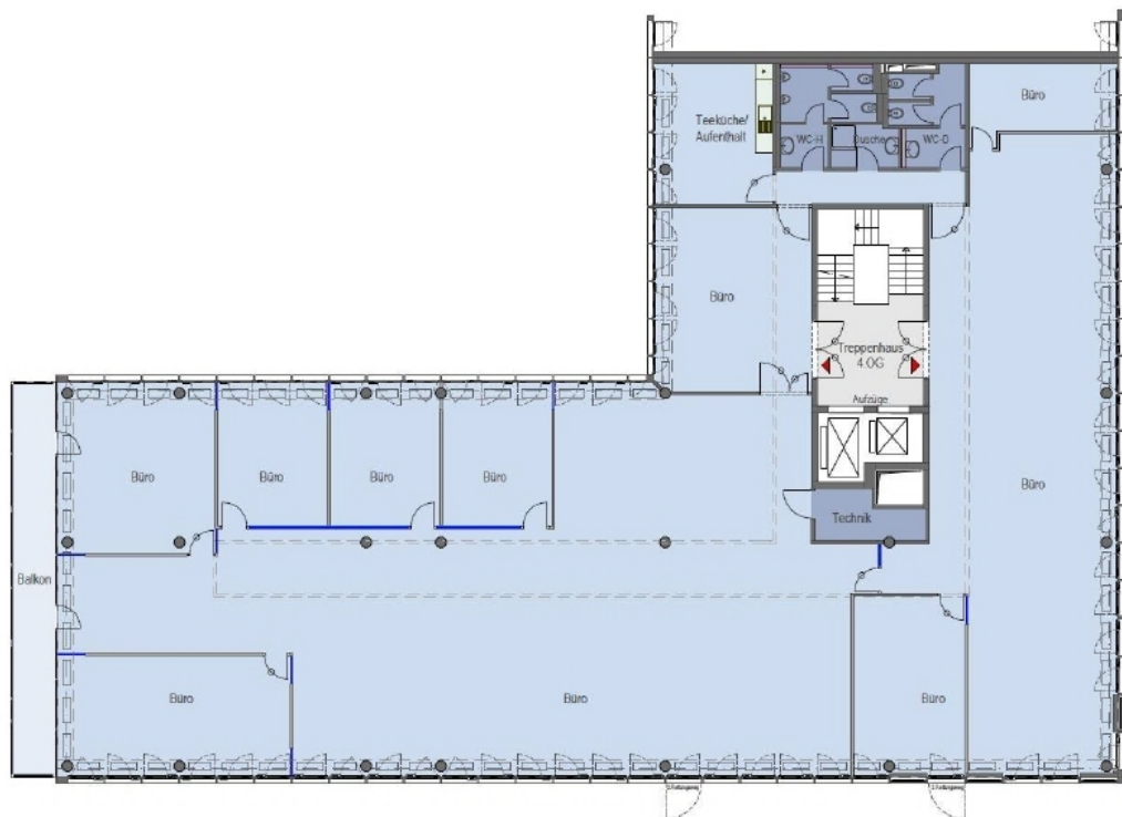
Grundriss 4OG
