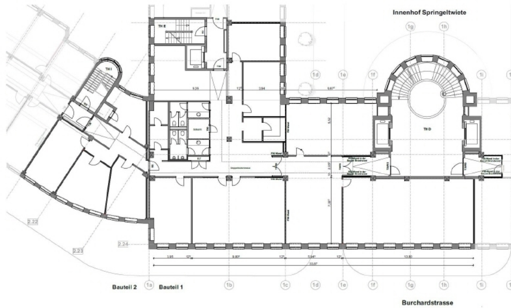
Grundriss 4 Obergeschoss
