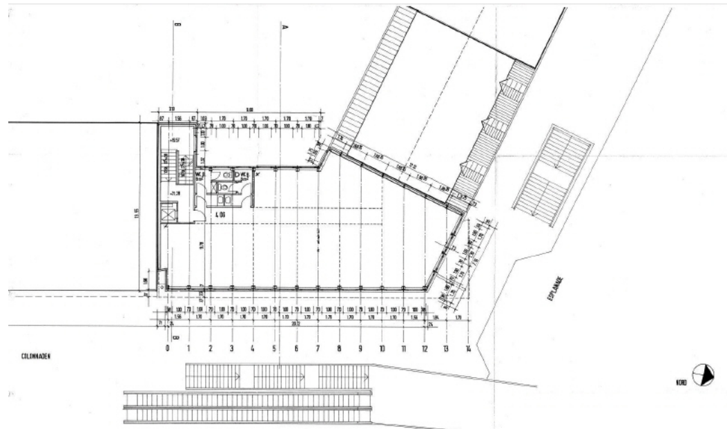
Grundriss 4.Obergeschoss
