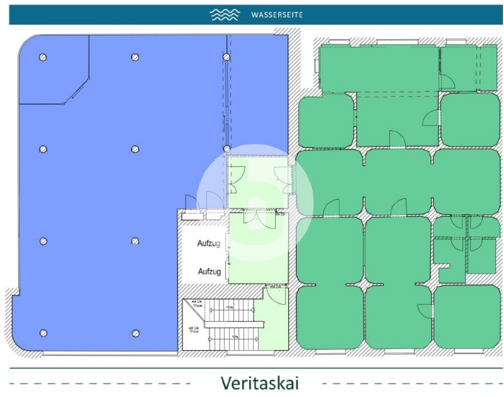
8 Obergeschoss mit ca 456 m 2
