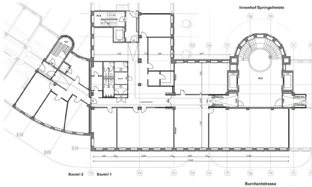
Grundriss 4 Obergeschoss
