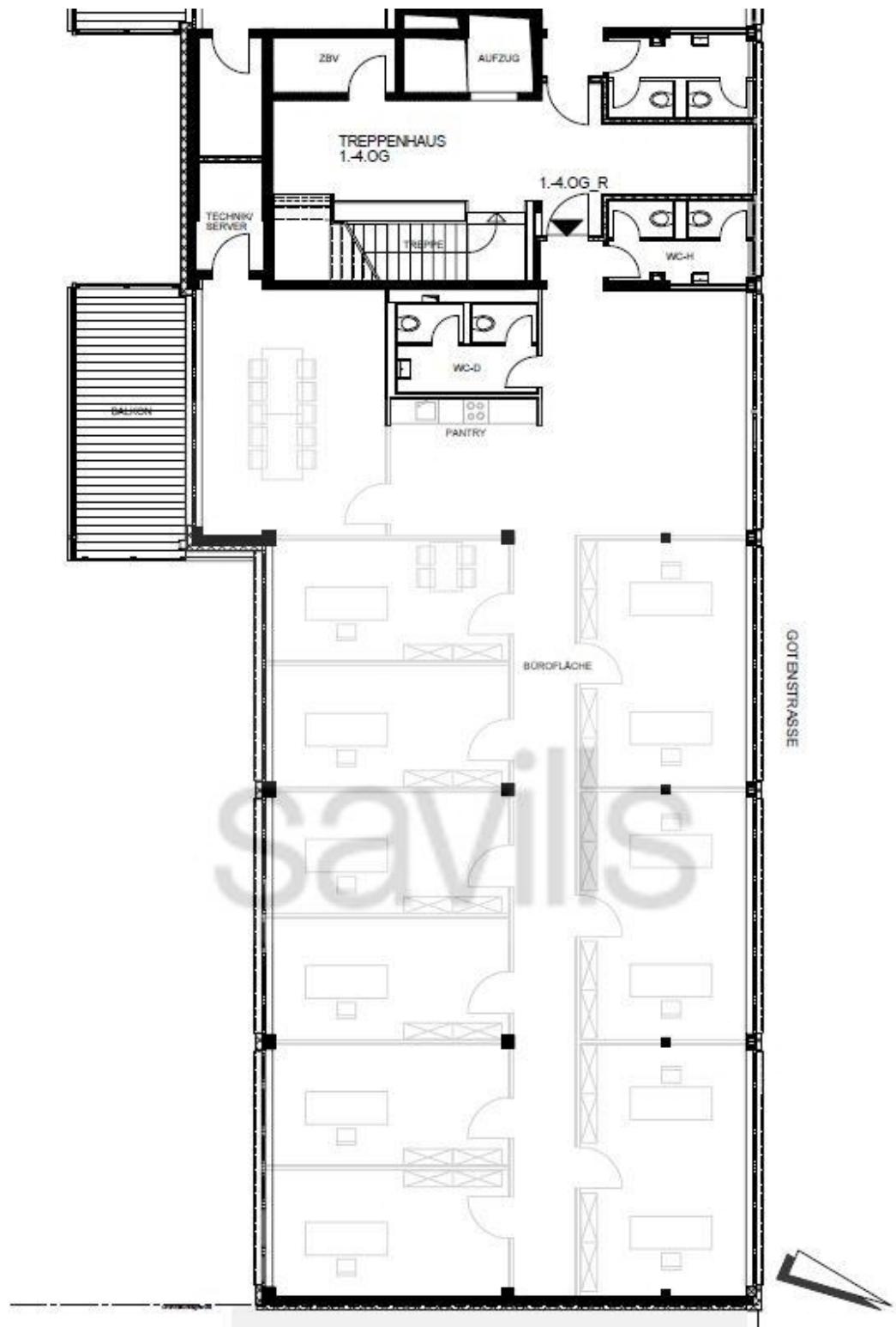
Grundriss, 4 OG, rechts ca 284,36 m 2
